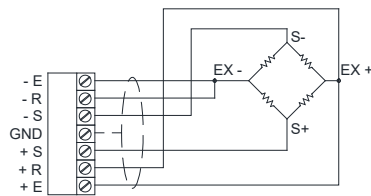
CONNEXION CAPTEURS À 6 FILS
