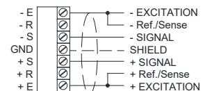
CÂBLE SORTIE À 6 FILS AVEC CAPTEUR À 4 FILS
